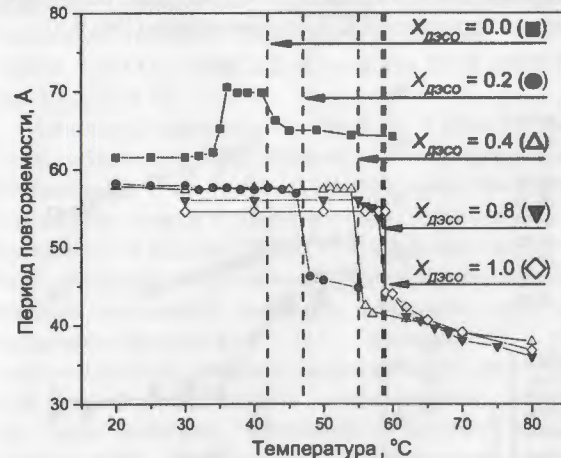
Рис.8. Зависимость периода повторяемости от температуры для МСВ ДПФХ (50 мас.%) для различных мольных долей ДЭСО в растворе ДЭСО/ H_2O . Вертикальные пунктирные линии соответствуют температурам основных фазовых переходов для соответствующих X_{DES} .
