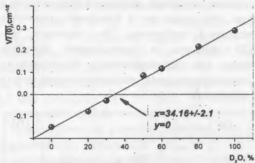
Рис.7. Зависимость \sqrt{I(0)} от процентного содержания D_2O для ОСВ ДМФХ (2 мас.%) в растворе ДМСО-d6/вода в гелевой фазе ( T = 15^\circ C ). Мольная доля ДМФХ-d6 X_{DMCO-d6} = 0.2 . Точка компенсации ( I(0) = 0 ) соответствует 34 % D_2O или \rho_{s,matching} = 3.53 \cdot 10^{10} \text{ см}^{-2} .
