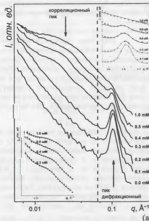
Рис.5. (а) – изменение кривых МУРН для МСВ ДМФХ (1 мас.%) в \text{D}_2\text{O} при добавлении ионов кальция; вертикальная пунктирная линия разграничивает области дифракционного и корреляционного пиков, аппроксимация которых функцией Гауссиана представлена линиями на вставках для экспериментальных данных (точки) для соответствующих концентраций; (б) – зависимость интегральной площади ( S_{\text{int}} ) и ширины ( w ) дифракционного пика от концентрации ионов кальция; (в) – зависимость периода повторяемости ( d ), корреляционной длины ( \xi ), определенных из аппроксимации дифракционного пика, и радиуса везикул ( R_v ), определенного из аппроксимации корреляционного пика, от концентрации ионов кальция.
