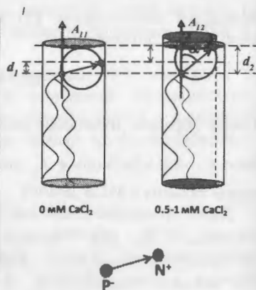
Рис.4. Схематичное изображение изменения направления P-N + диполя в ЖК фазе: слева – ОСВ ДМФХ (1 мас.%) в \text{D}_2\text{O} ; справа – ОСВ ДМФХ (1 мас.%) в растворе \text{CaCl}_2 \cdot 2\text{H}_2\text{O}/\text{D}_2\text{O} , полученных из МСВ.
