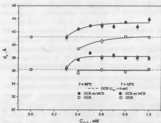
Рис.3. Зависимость толщины липидного бислоя от концентрации ионов кальция для МСВ ДМФХ (1 мас.%) в растворе \text{CaCl}_2 \cdot 2\text{H}_2\text{O}/\text{D}_2\text{O} (серия А-I) и ОСВ ДМФХ (1 мас.%) в гелевой ( T = 15^\circ\text{C} ) и ЖК ( T = 55^\circ\text{C} ) фазах.
