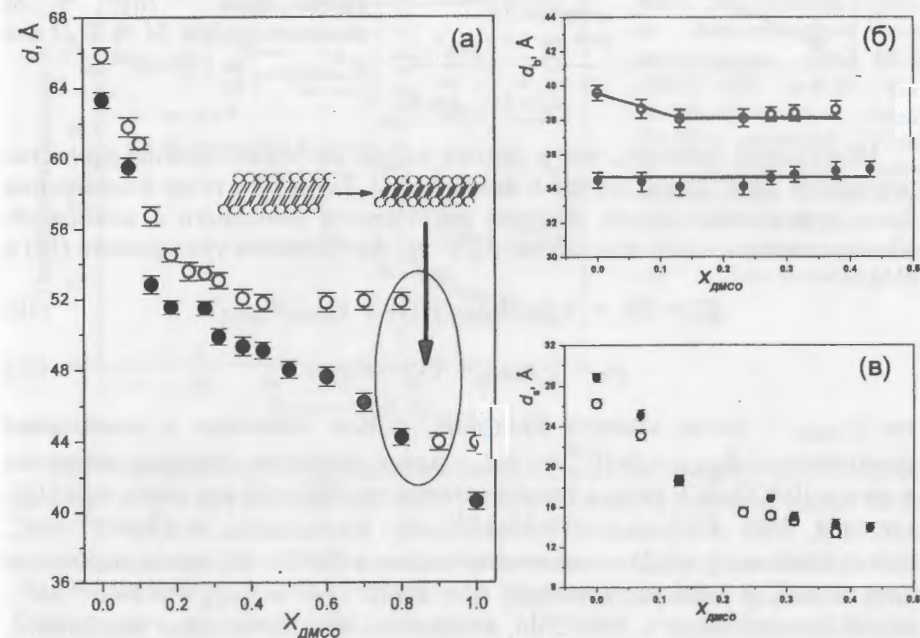
Рис.6. Зависимости (а) периода повторяемости d , (б) толщины липидного бислоя d_b и (в) межмембранного расстояния d_s = d - d_b от мольной доли ДМСО для ДМФХ-d54 мембран (2 мас.%) в растворе ДМСО/вода в гелевой ( T = 12.5 °C) и ЖК ( T = 55 °C) фазах. Открытые и закрашенные круги соответствуют гелевой и ЖК фазам.
