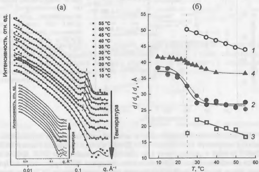
Рис.9. (а) - Изменение кривых МУРН для ОСВ ДМФХ (2 мас. %) в D_2O после добавления ДЭСО ( X_{\text{ДЭСО}} = 0.1 ) и стабилизации в течение 3 ч при T = 55^\circ\text{C} при охлаждении от 55 до 10^\circ\text{C} и нагревании от 10 до 55^\circ\text{C} (вставка). Пунктирной линией показано изменение положения q_0 ; (б) - Температурная зависимость структурных параметров системы, полученной для ОСВ ДМФХ (2 мас. %) в D_2O после добавления ДЭСО ( X_{\text{ДЭСО}} = 0.1 ): периода повторяемости МСВ d (1); толщины липидного бислоя d_b (2); межмембранного расстояния d_s (3); толщины липидного бислоя ОСВ ДМФХ (2 мас. %) в D_2O (4). Черные символы - нагревание, серые символы - охлаждение. Линии - аппроксимация функцией (10) параметра d_b и прямых параметров d и d_s . Вертикальная пунктирная линия обозначает температуру основного фазового перехода для ОСВ ДМФХ (2 мас. %) в D_2O при добавлении ДЭСО ( X_{\text{ДЭСО}} = 0.1 ).
